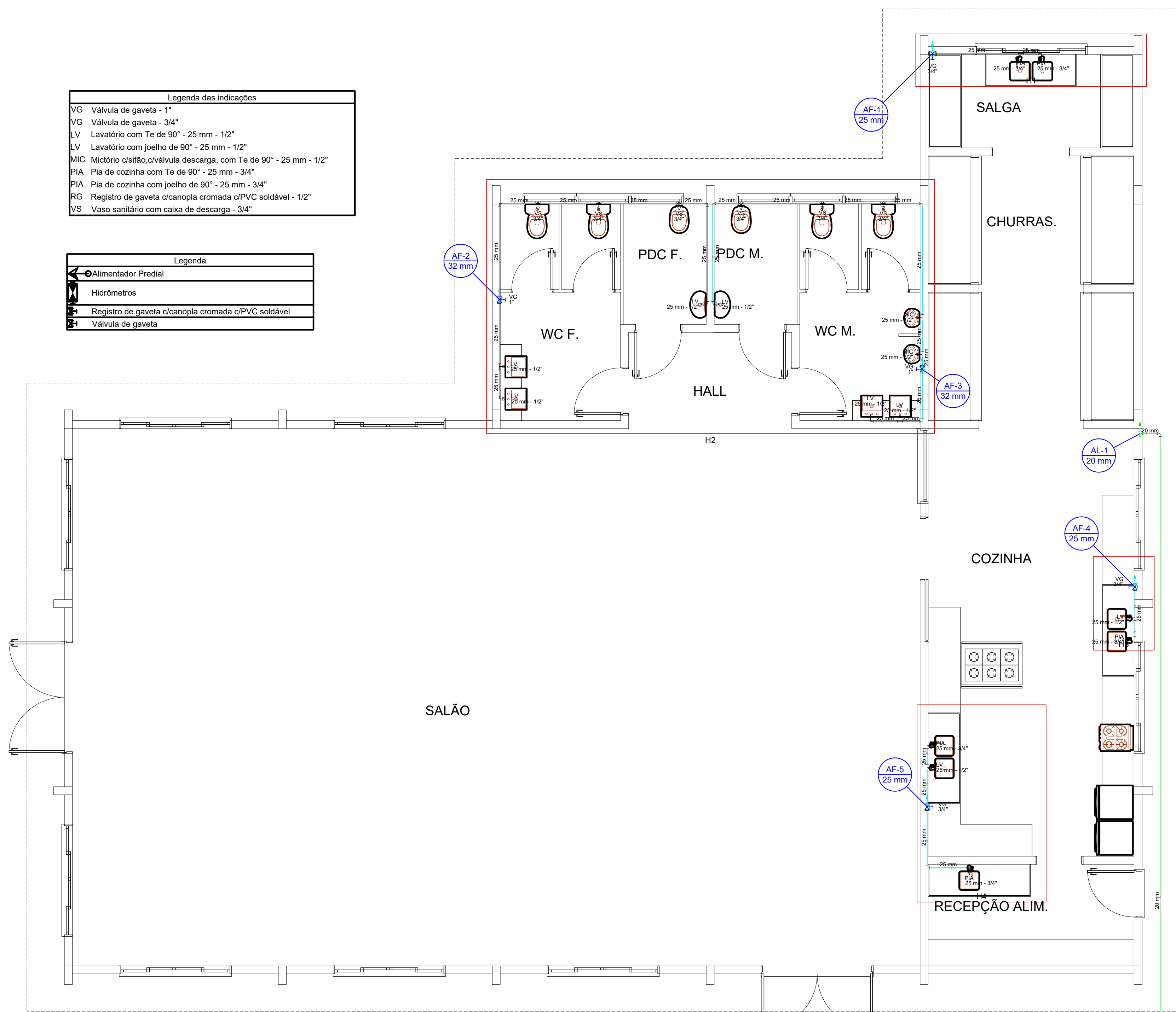
PLANTA BAIXA HIDRÁULICA PAVIMENTO INFERIOR Área: 312,80 m² Escala: 1:50
