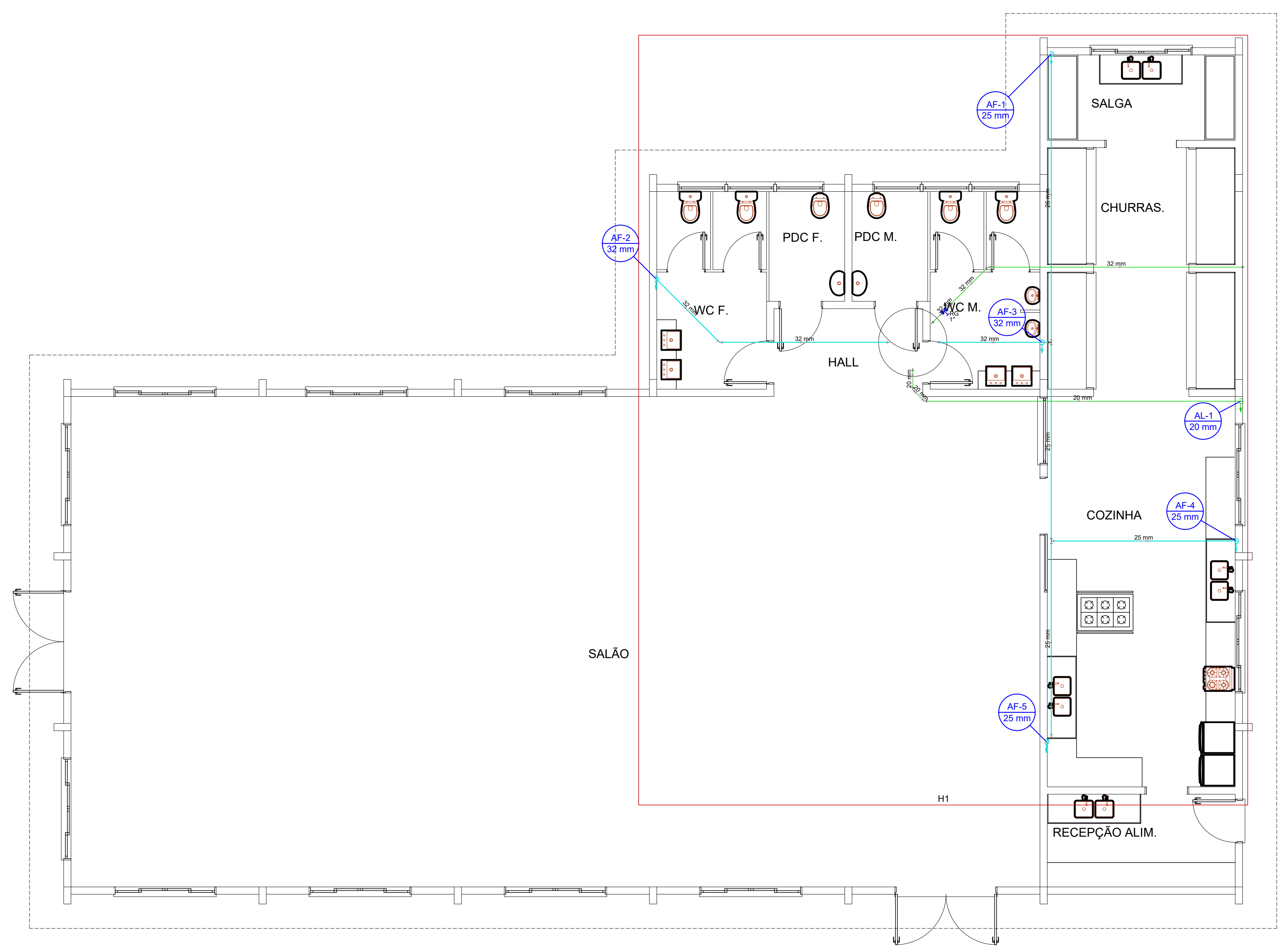
PLANTA BAIXA HIDRÁULICA PAVIMENTO INFERIOR Área: 312,80 m² Escala: 1:50
