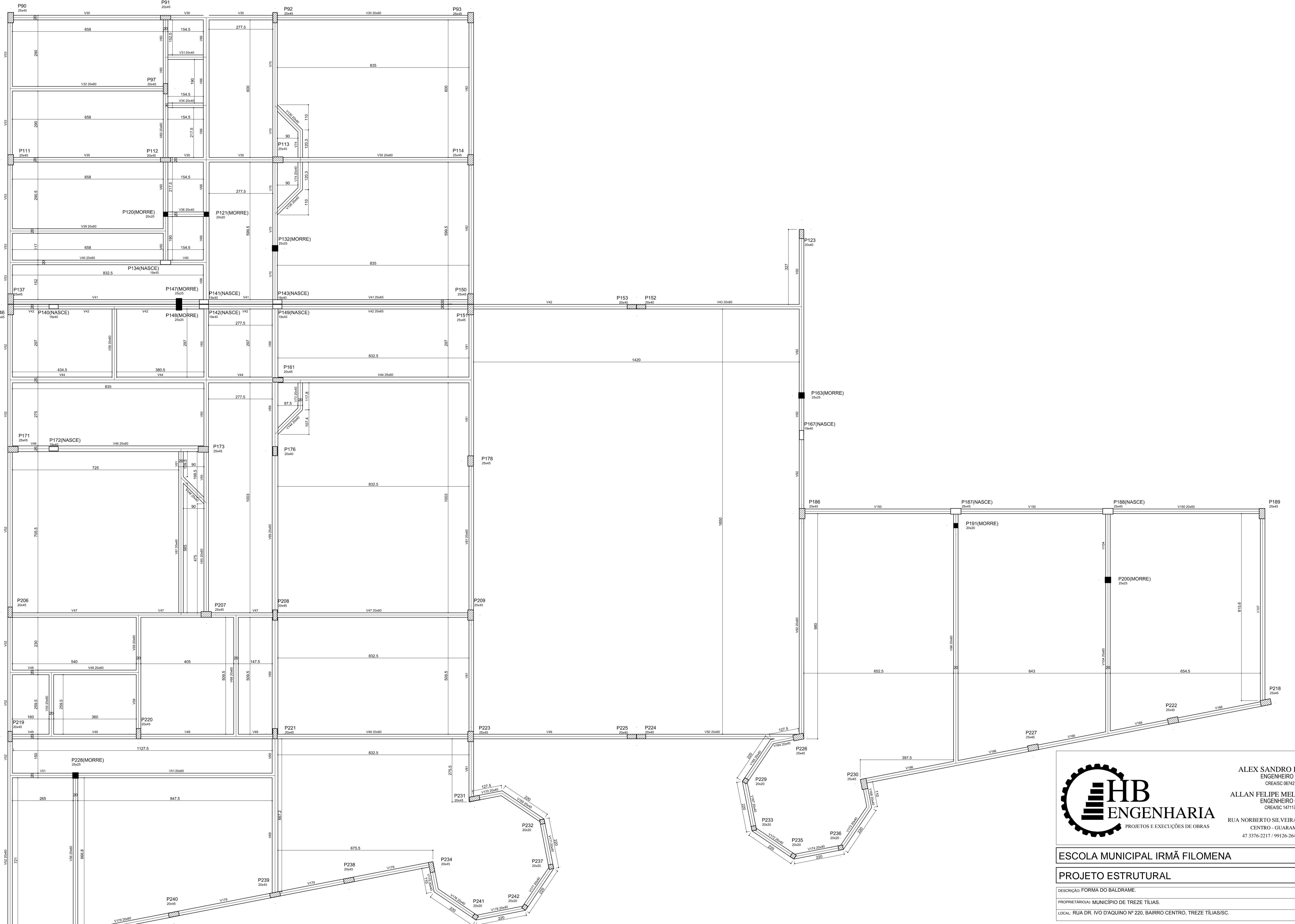
Forma do baldrame escala 1:75
