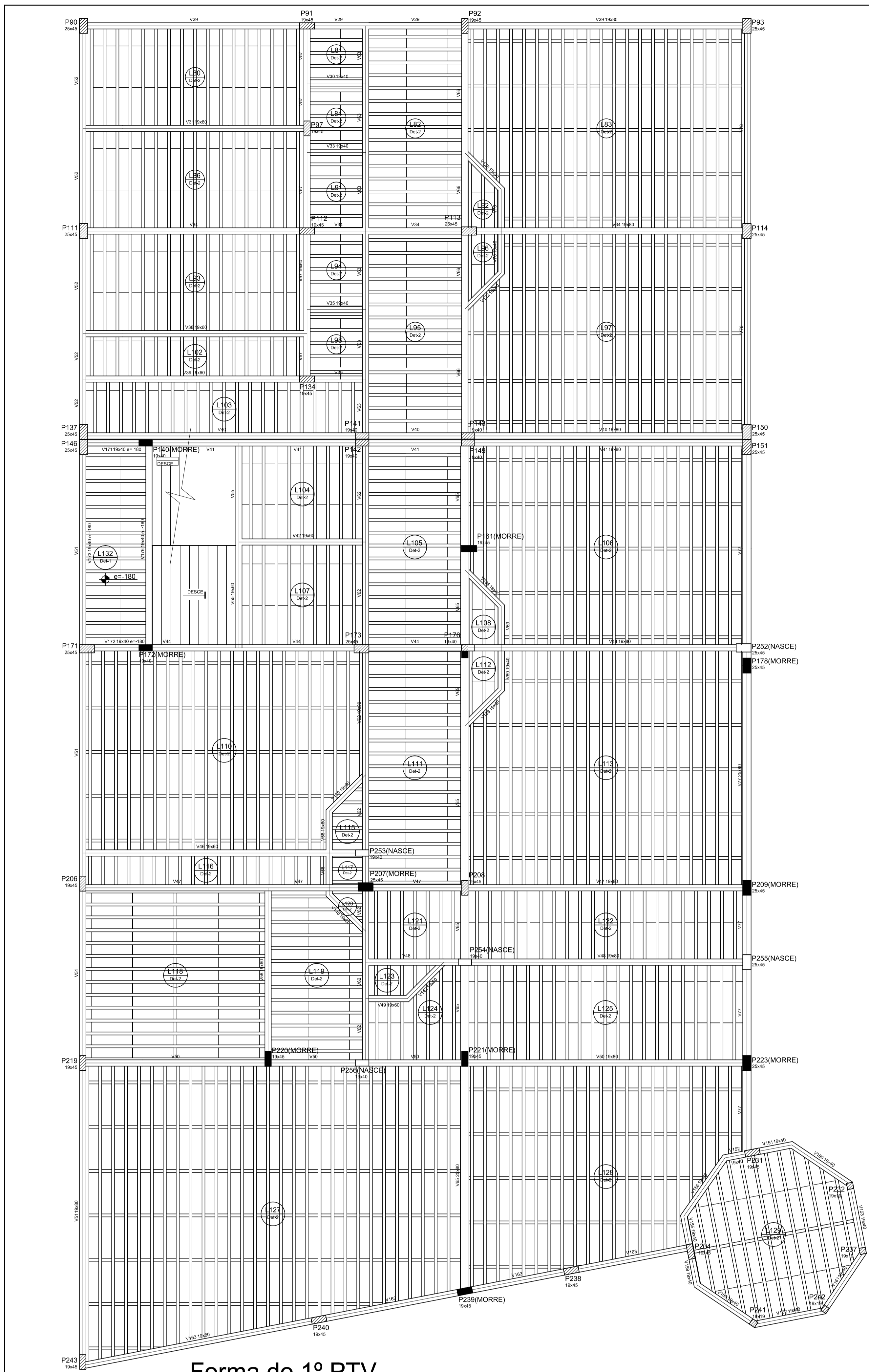
Forma do 1º PTV escala 1:75
