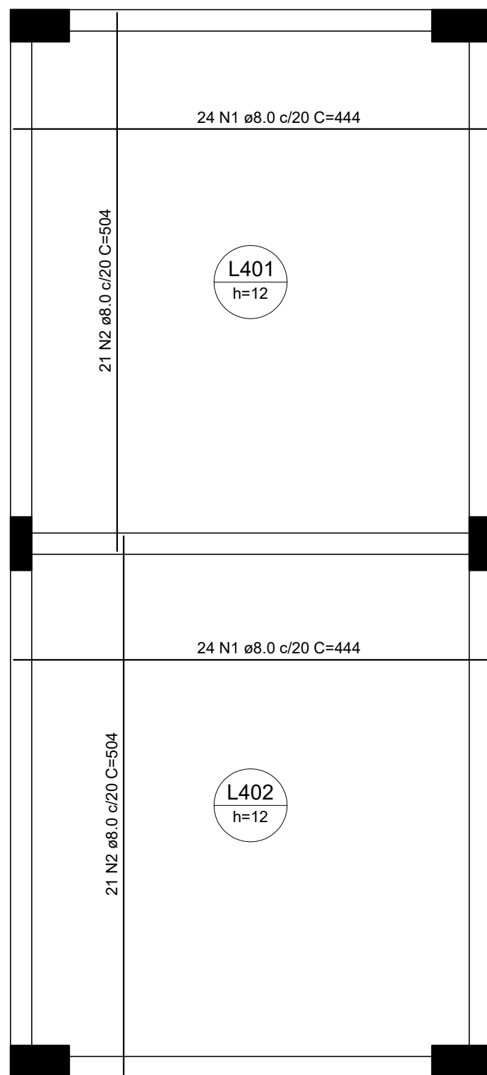
Armação positiva das lajes do pavimento Cobertura
