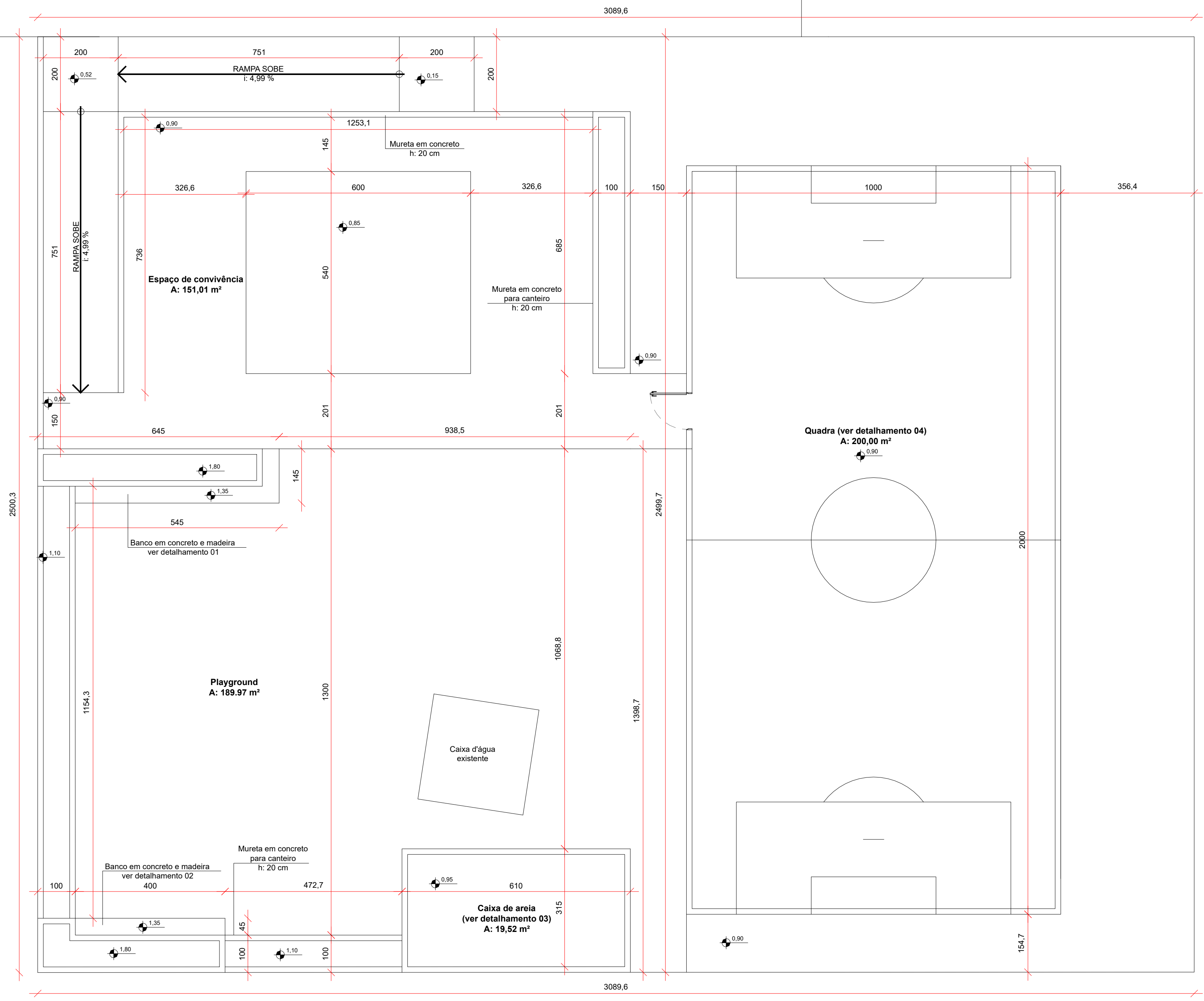
Planta baixa - Técnica Esc: 1/75 Área: 772,32 m²
