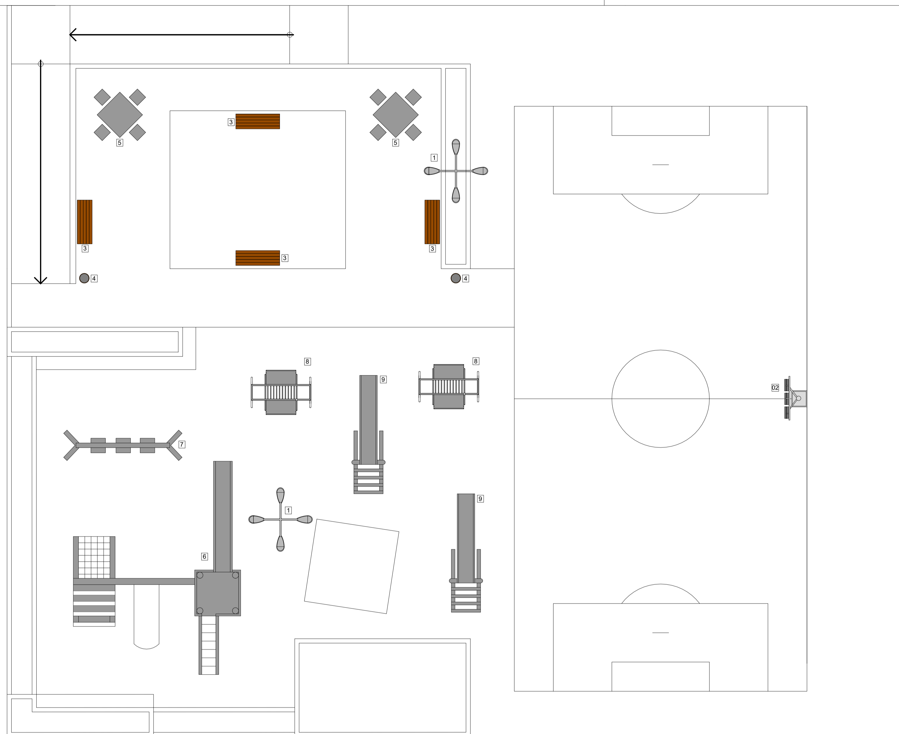
Planta baixa - Mobiliário Urbano Esc: 1/75
