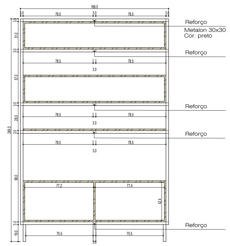
Corte AA
