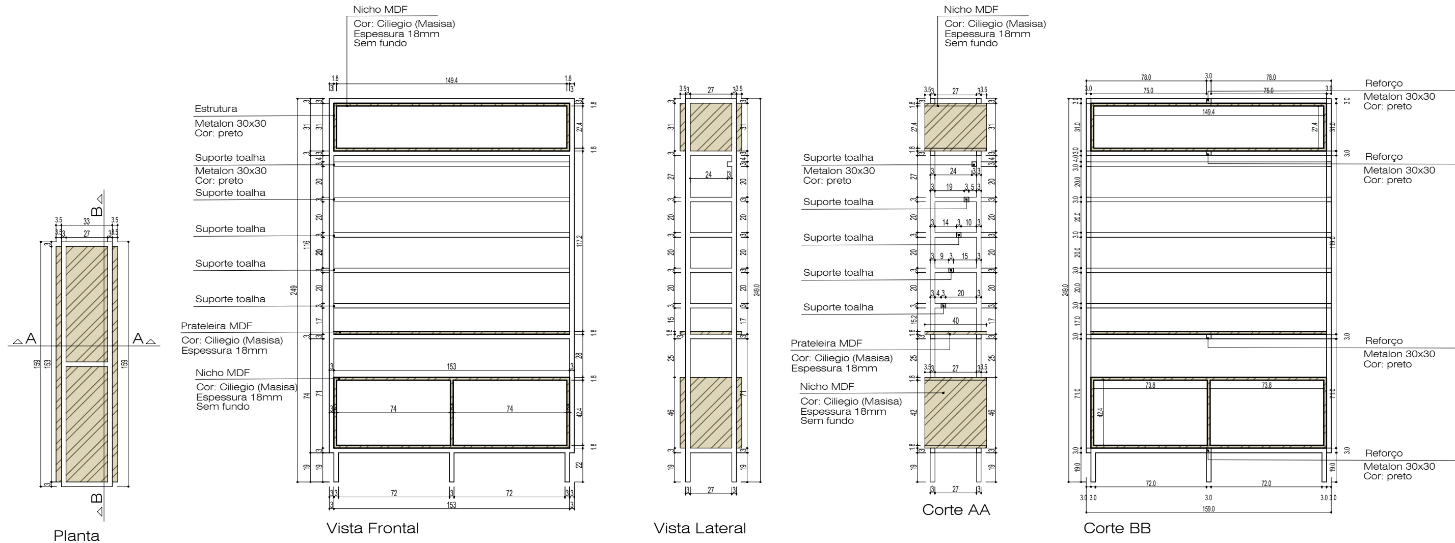
12 Detalhe 06 Esc: 1/25
