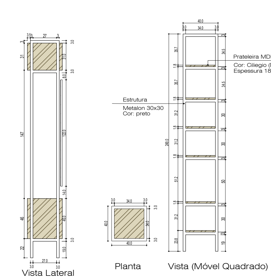
21 Detalhe 11 Esc: 1/25
