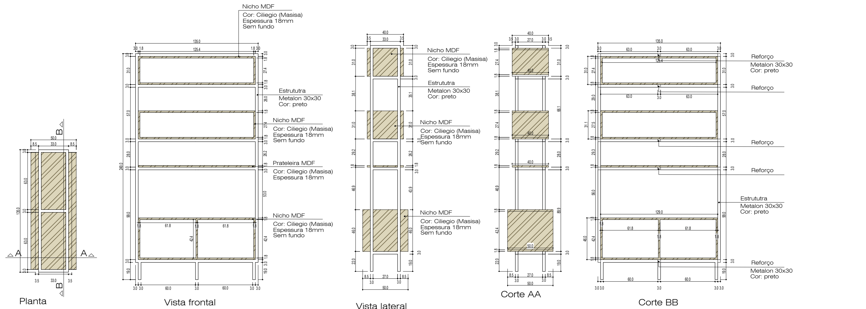
26 Detalhe 13 Esc: 1/25
