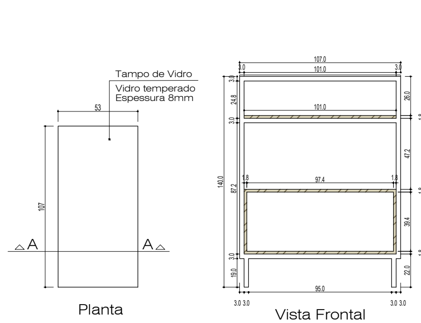
40 Detalhe 18 Esc: 1/25
