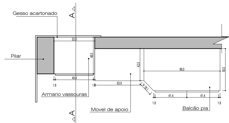
Em planta
