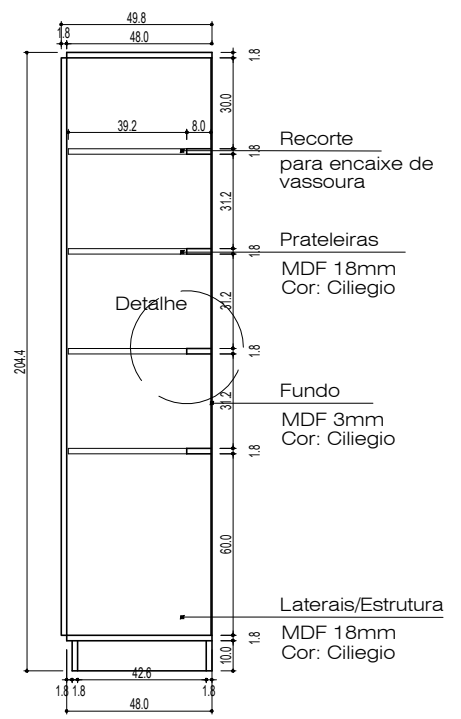
Corte AA Armário de vassouras
