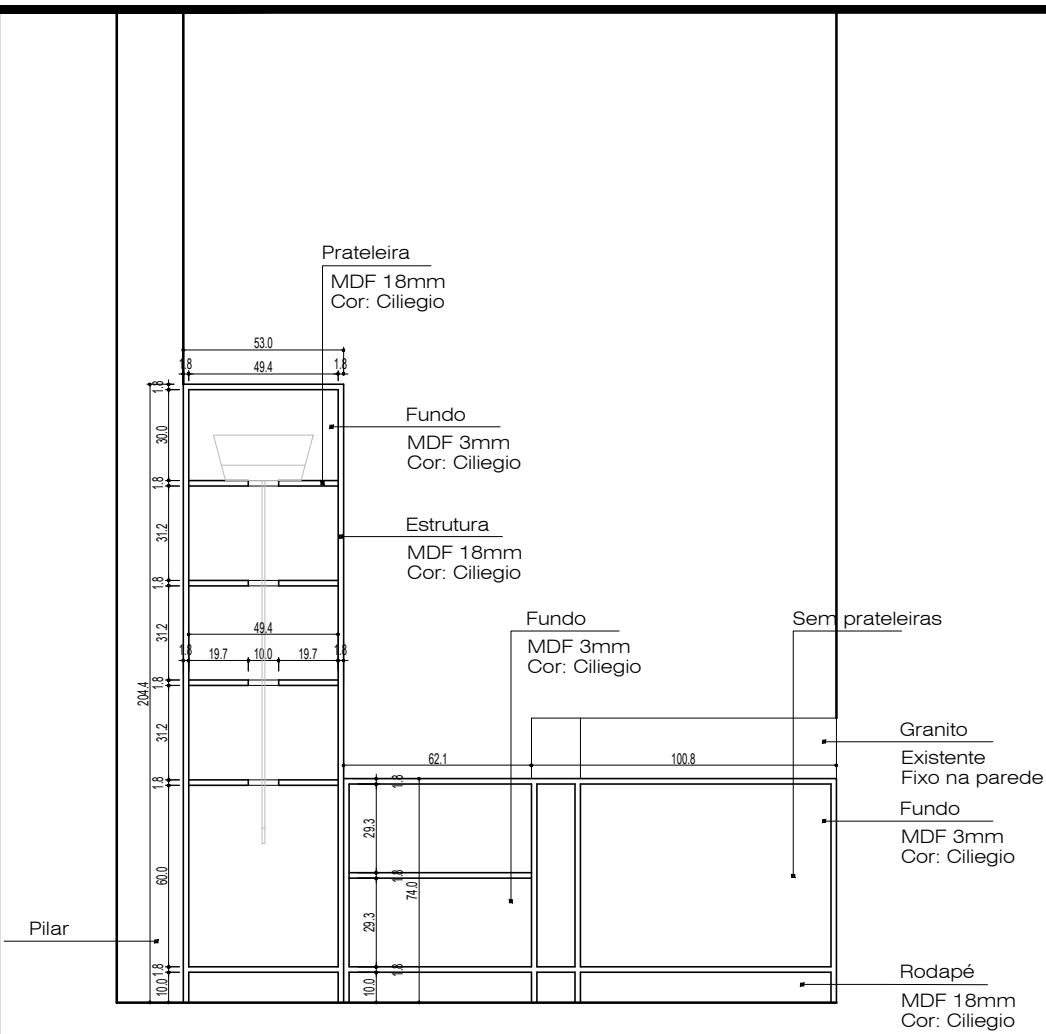
Vista frontal (sem portas)
