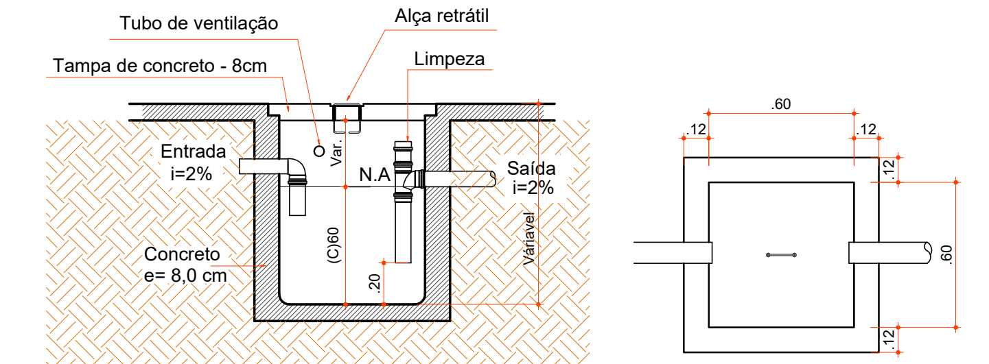
DETALHE CAIXA DE GORDURA Escala 1:25
