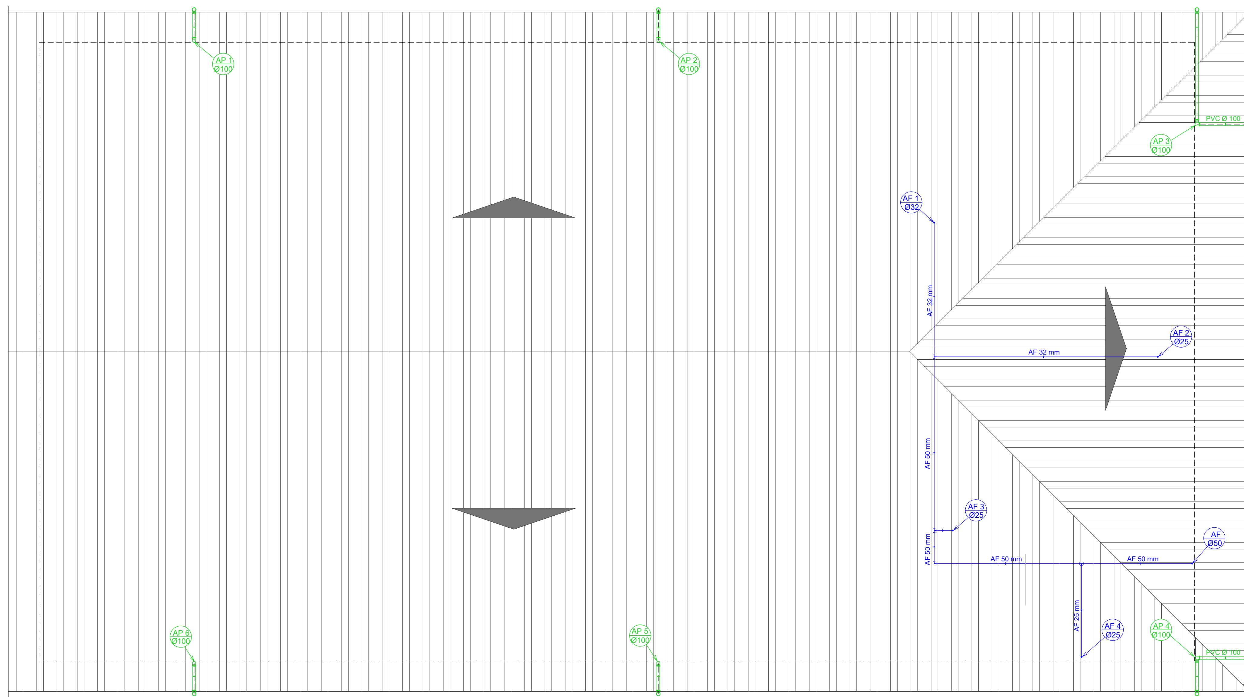
PLANTA DE COBERTURA Escala 1:75
