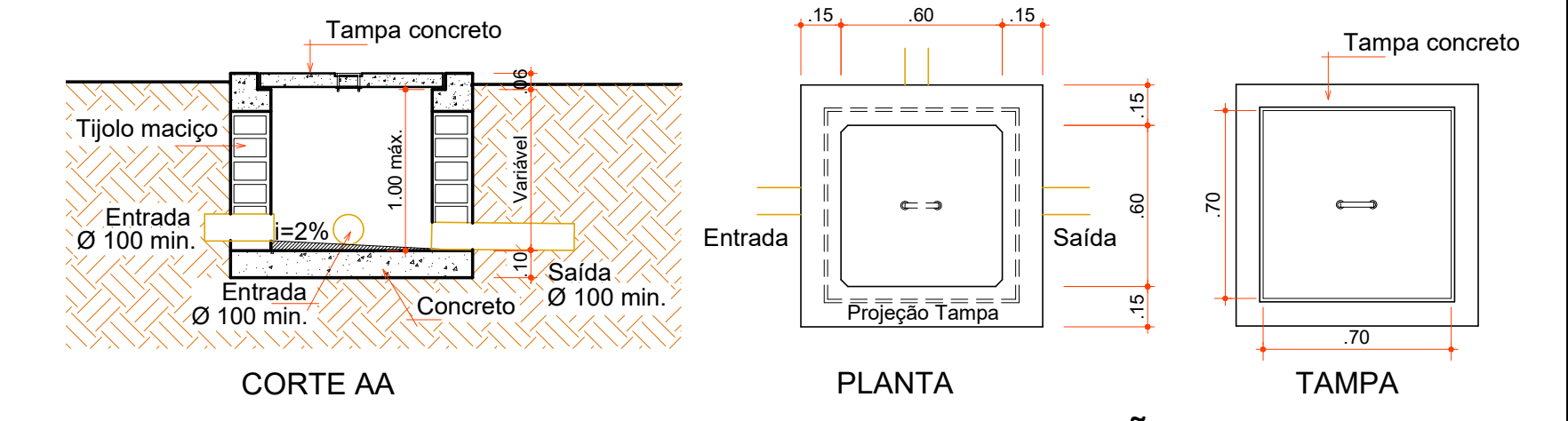
DETALHE CAIXA DE INSPEÇÃO Escala 1:25
