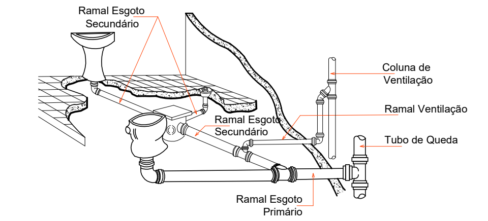
DETALHE COLUNA DE VENTILAÇÃO Escala 1:33
