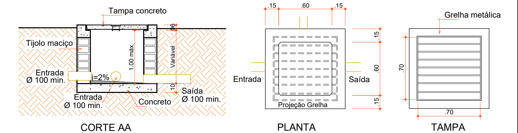
DETALHE CAIXA DE PASSAGEM Escala 1:25
