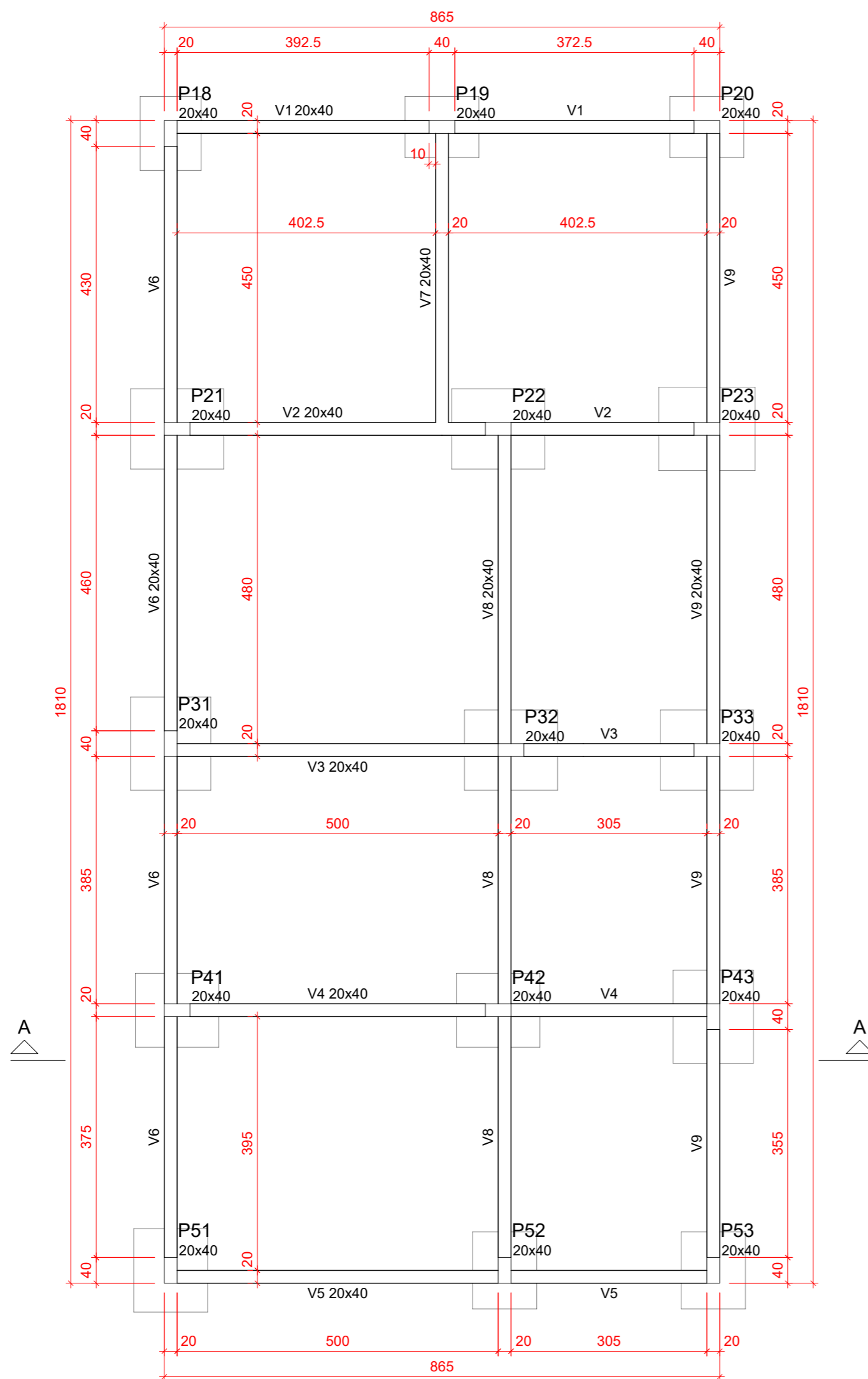
Planta de Formas do Pilotis (Nível -250) escala 1:75
