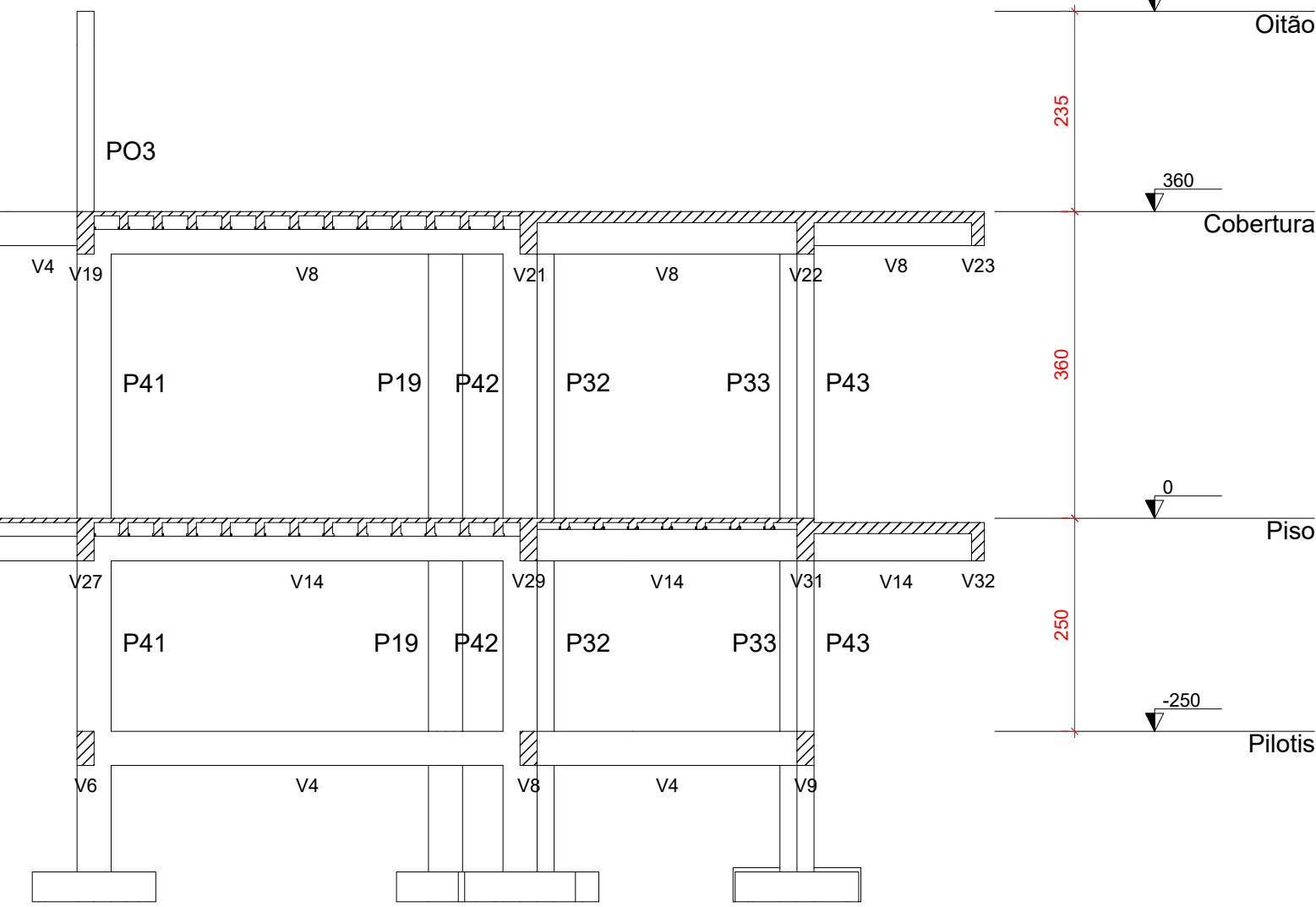
Corte A-A escala 1:75
