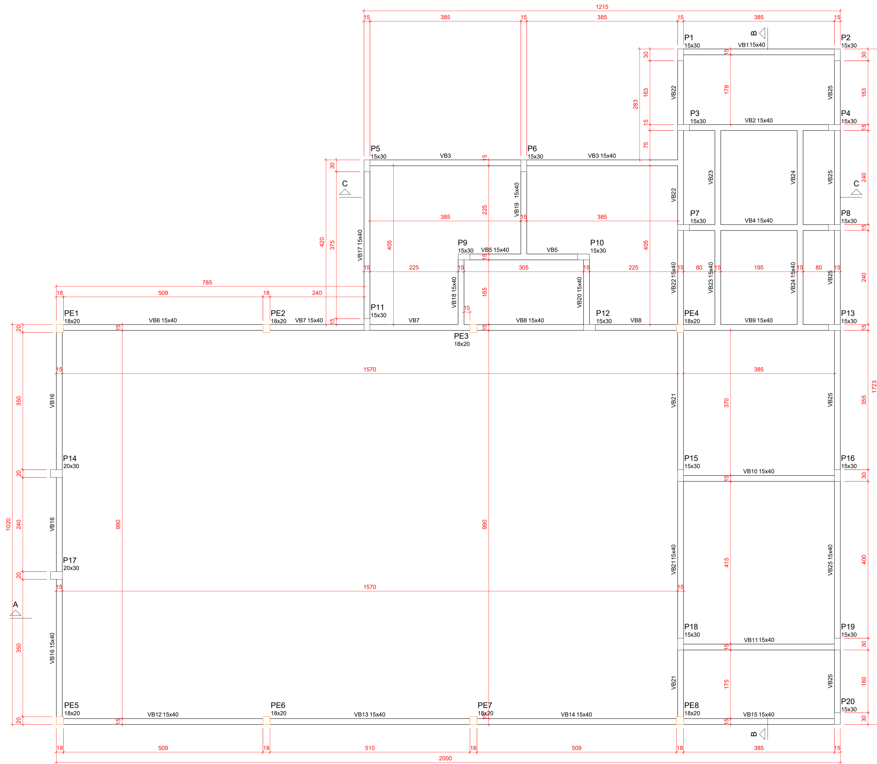
Planta de Formas do Baldrame (Nível 0) escala 1:50
